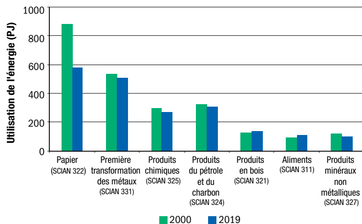
Figure 3. Consommation d'énergie dans les sept sous-secteurs sélectionnés, 2000 et 2019
