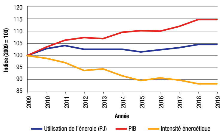
Figure 1. Indice de croissance de l'utilisation de l'énergie, du PIB et de l'intensité énergétique dans le secteur manufacturier, 2009-2019
