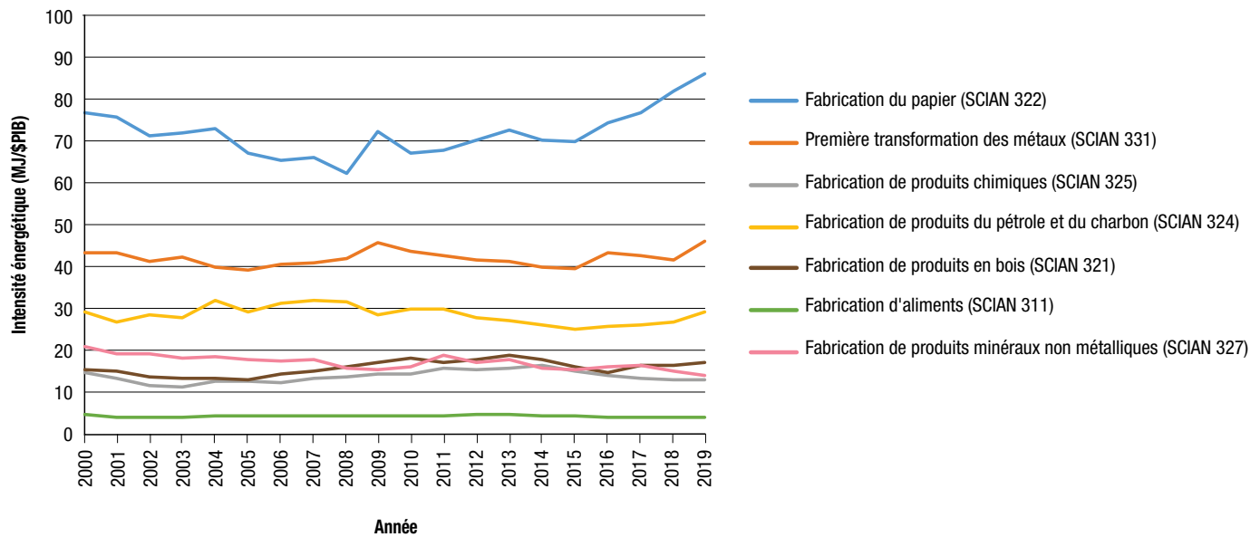
Figure 2. Intensité énergétique dans les sept sous-secteurs sélectionnés, de 2000 à 2019
